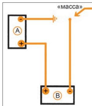
Рис. 24. Схема подключения вспомогательной батареи
