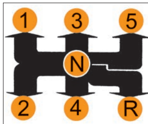
Рис. 22. Схема переключения передач
