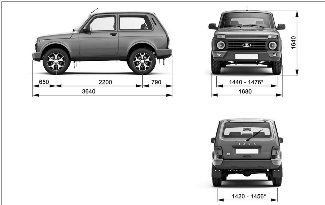
Рис. 54. Габаритные размеры автомобиля LADA Niva Legend Urban 3 дв.
