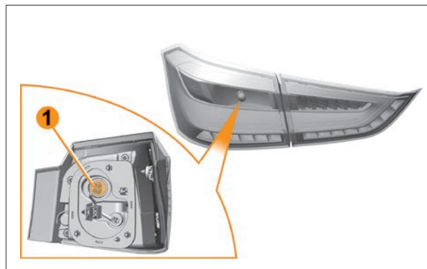
Рис. 6.12.1. Лампа указателя поворота в заднем фонаре
